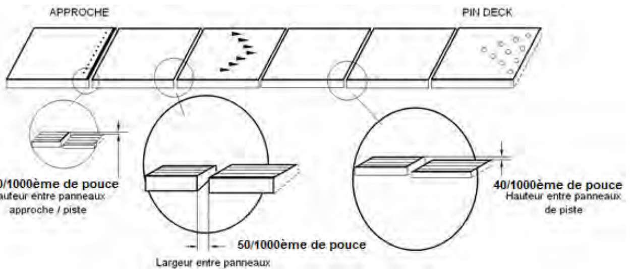
Figure 5 – Ajustement des panneaux de piste
